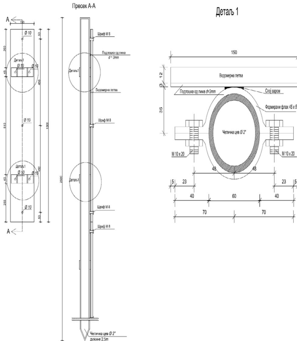
Носач челични цевасти са основом Радионички цртеж подлошке за водомерну летву
