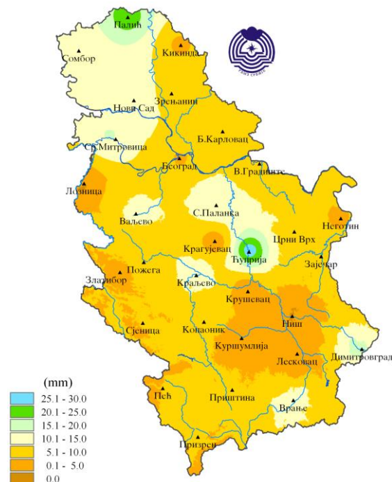
Слика 2. Количина падавина за период 17–24.6.2022. године
