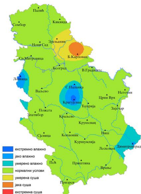
Слика 3. Услови влажности у Србији, процењени на основу Стандардизованог падавинског индекса (SPI-1) одређеног за временски период од 30 дана (25.05 – 23.06.2022. године)
