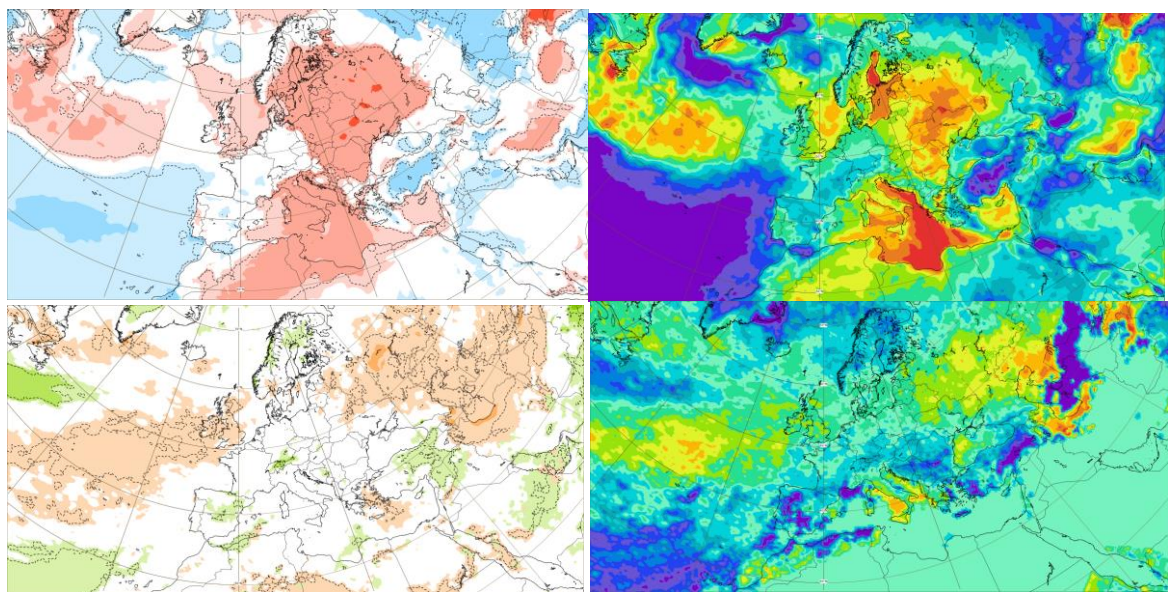
Слика 6. Прогноза одступања средње недељне температуре ваздуха и вероватноћа за горњи терцил (први ред) и суфицита/дефицита падавина и вероватноћа за доњи терцил (други ред) за период од 4.7. до 11.7.2022.
