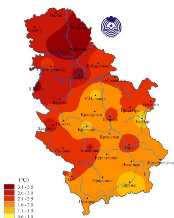
Слика 1. Одступање средње температуре ваздуха од нормале 1981–2010. године за период 17–24.6.2022. године
