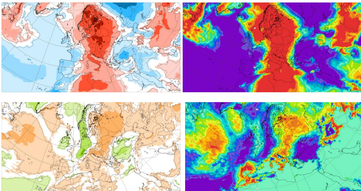
Слика 5. Прогноза одступања средње недељне температуре ваздуха и вероватноћа за горњи терцил (први ред) и суфицита/дефицита падавина и вероватноћа за доњи терцил (други ред) за период од 27.6. до 4.7.2022.
