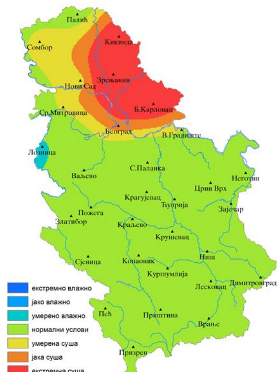
Слика 4. Прогноза Стандардизованог падавинског индекса одређеног за временски период од 30 дана (SPI-1) рађена на основу осматраних и Прогнозираних падавина (04.06–03.07.2022. године) Европског центра за средњорочну прогнозу времена и Републичког хидрометеоролошког завода.
