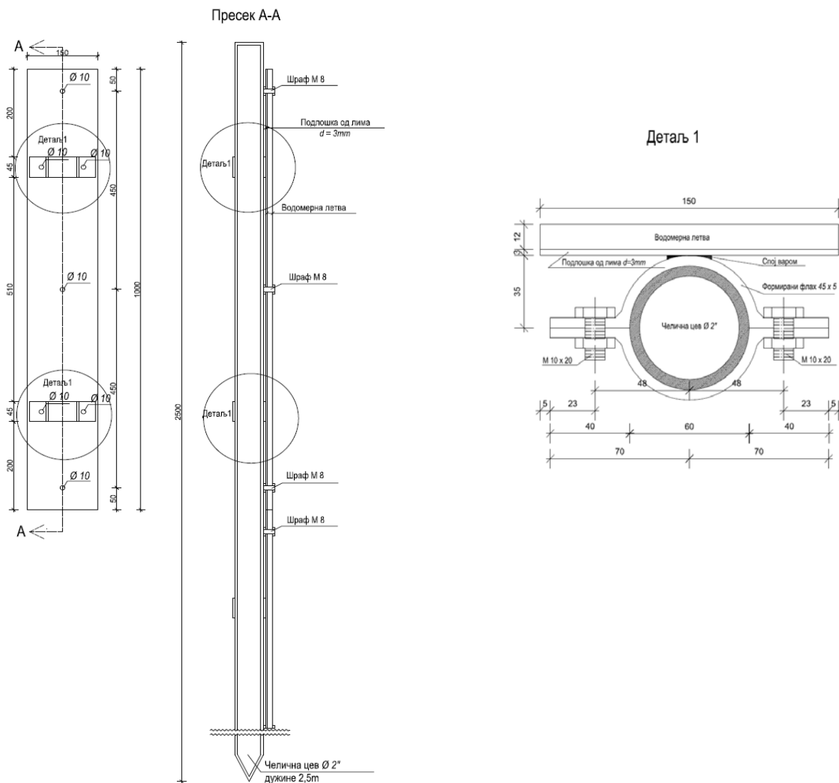
Носач челични цевасти са основом Радионички цртеж подлошке за водомерну летву
